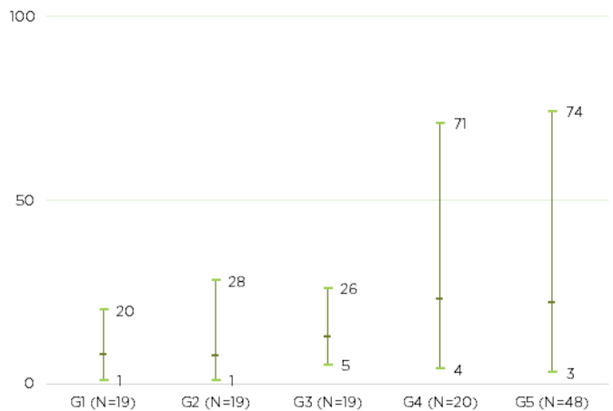
Figura 10. Número de categorías comerciales. Se muestran máximos, mínimos y promedio para cada estrato de población.
